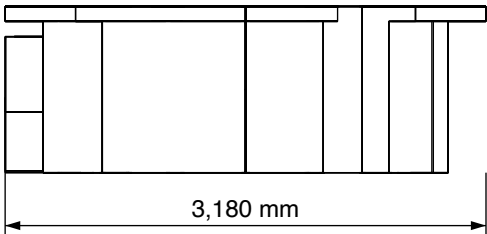
VISTA LATERAL
